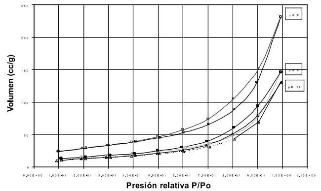
Fig. 2- Isotermas de Adsorción para el nanocompuesto CdS.
